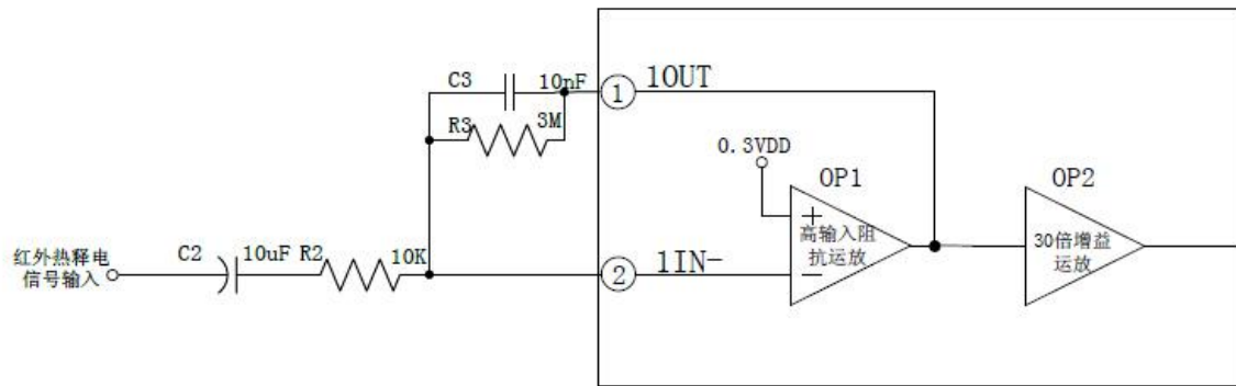
图 8.5a DL7955 内部运放框图
