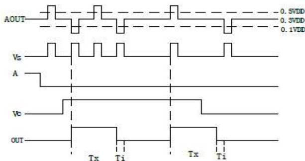
图 8.3a 不可重复触发工作方式波形
