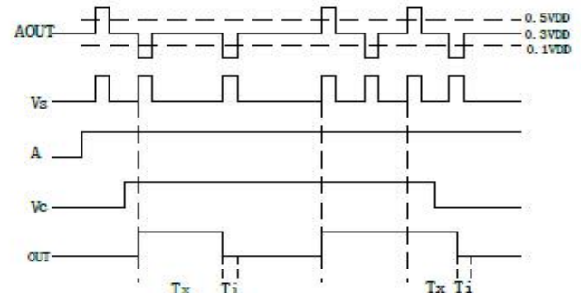
图 8.3b 可重复触发工作方式波形
